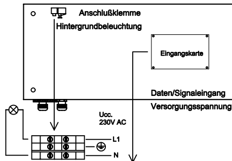
Innenansicht - Anschlussklemmen
